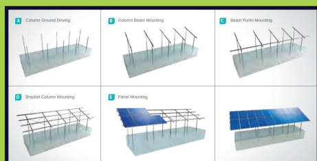
Sistema de Montaje en Acero para Suelo con 2 Paneles Verticales
