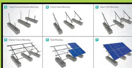
Sistema de Montaje en Acero Anclado en Base de Concreto con 2 Paneles Verticales
